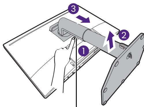
Кнопка разъединения
